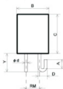
Technická specifikace nástroje pro tvarování Typu A
